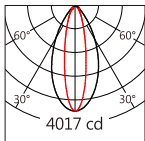
3030 25°X45° 4000K
