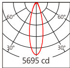
3030 30° 3000K
